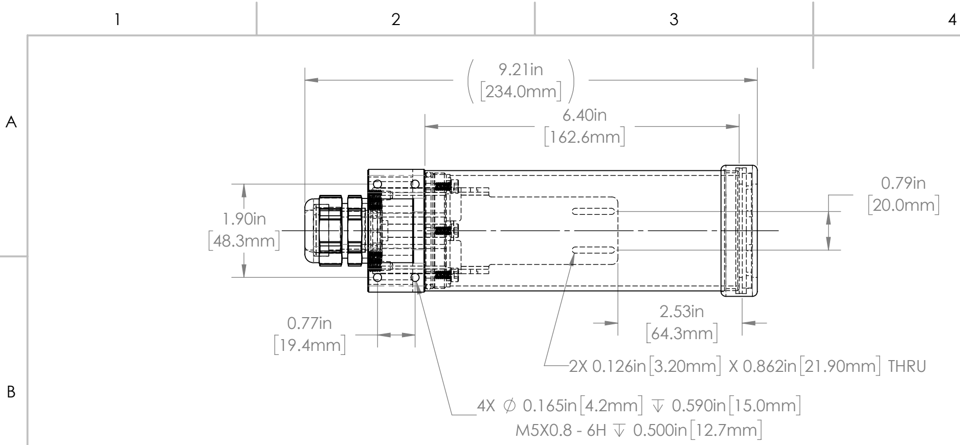
SECTION A-A
