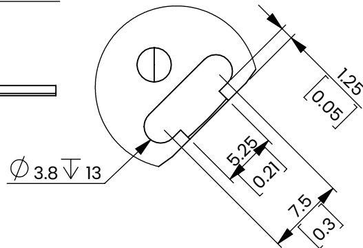
T-Slot DETAIL A SCALE 2:1 (2:1)
